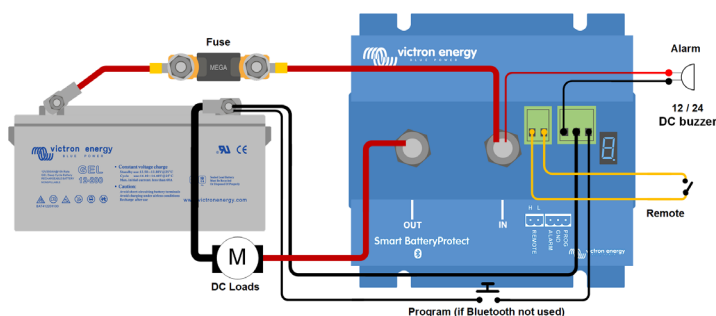
Kontakt med förmonterad DC-minuskabel (ingår)
